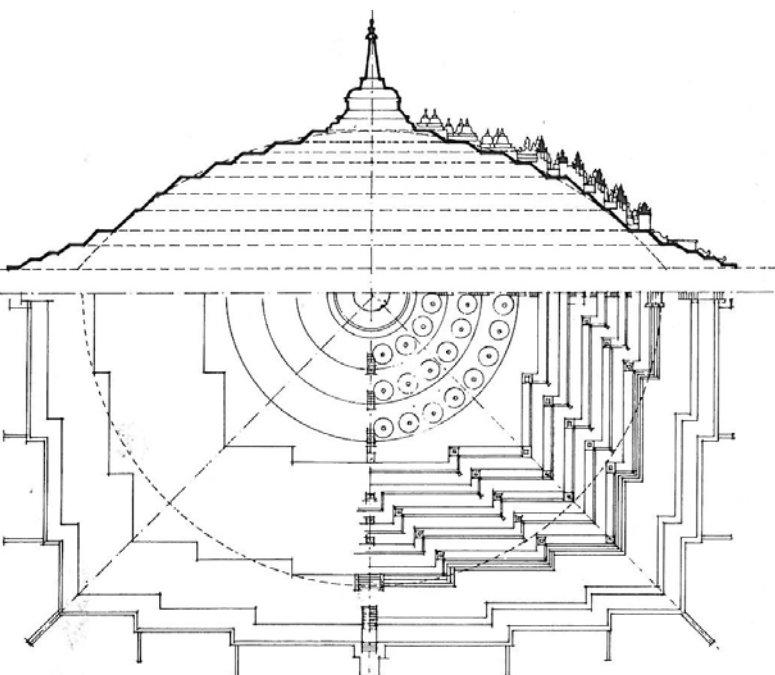
Borobudur, plan og snitt. Tegning: Sestini og Somigli : Sherpa architecture ,Unesco 1978
