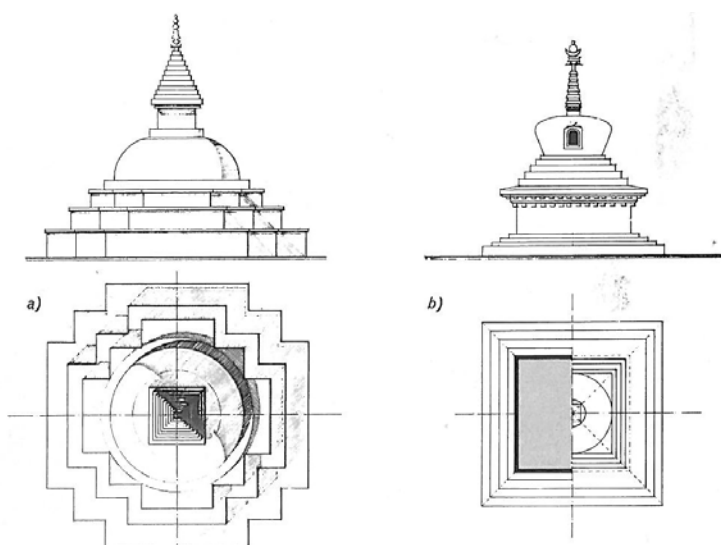
Stupa, chorten. Tegning: Sestini og Somigli : Sherpa architecture ,Unesco 1978
